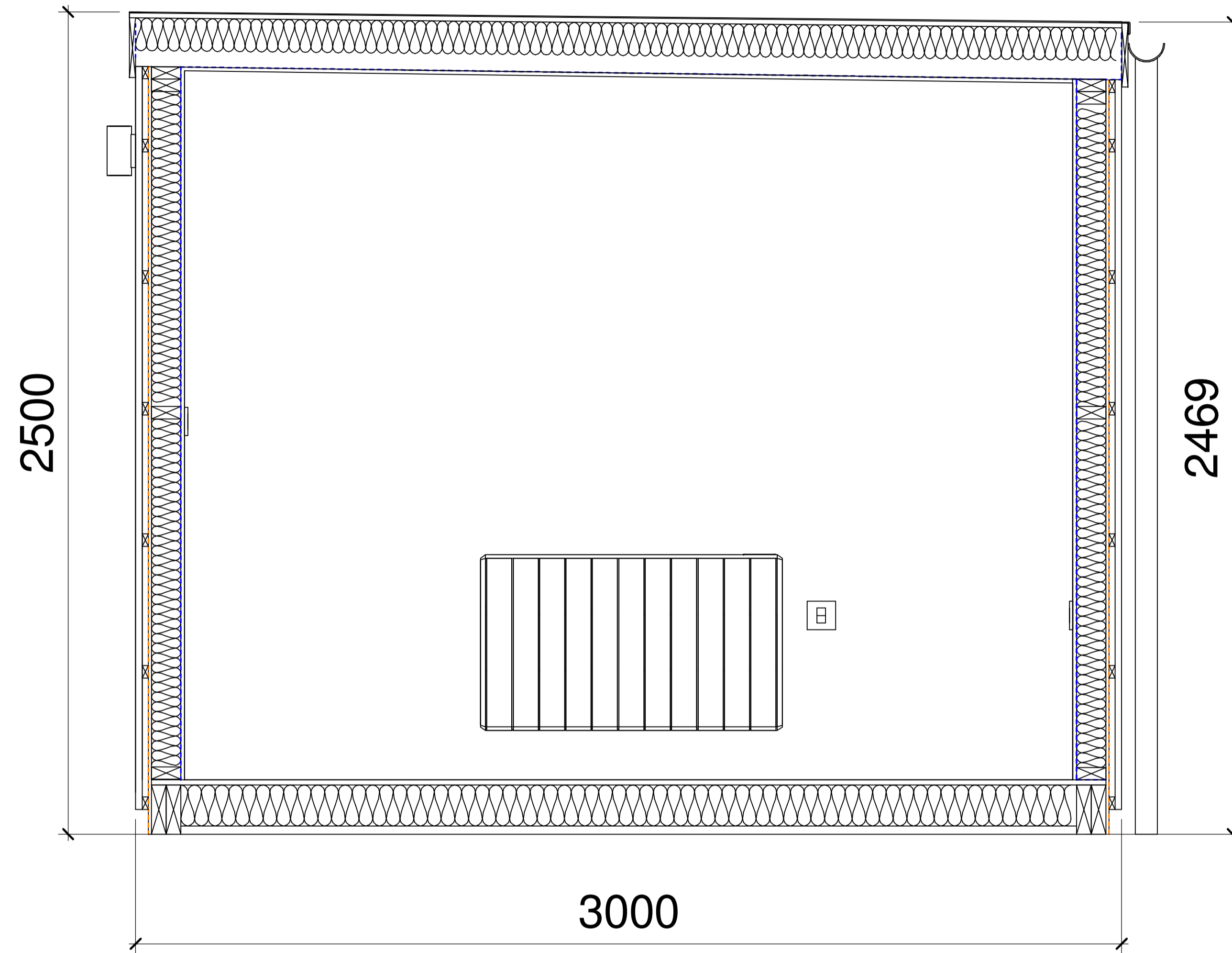
2 Section Type 2 1 : 20
